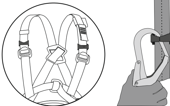
Рис. 5. Правильная установка скобы на ленте
