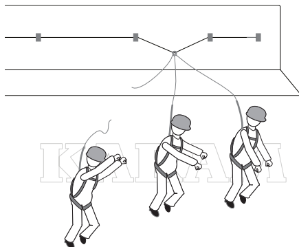
Рис. 4. Фактор перерезания
