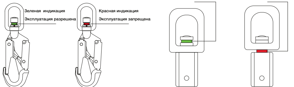
Рис. 6. Индикаторы срабатывания
