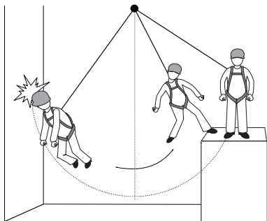
Рис. 3. Фактор маятника
