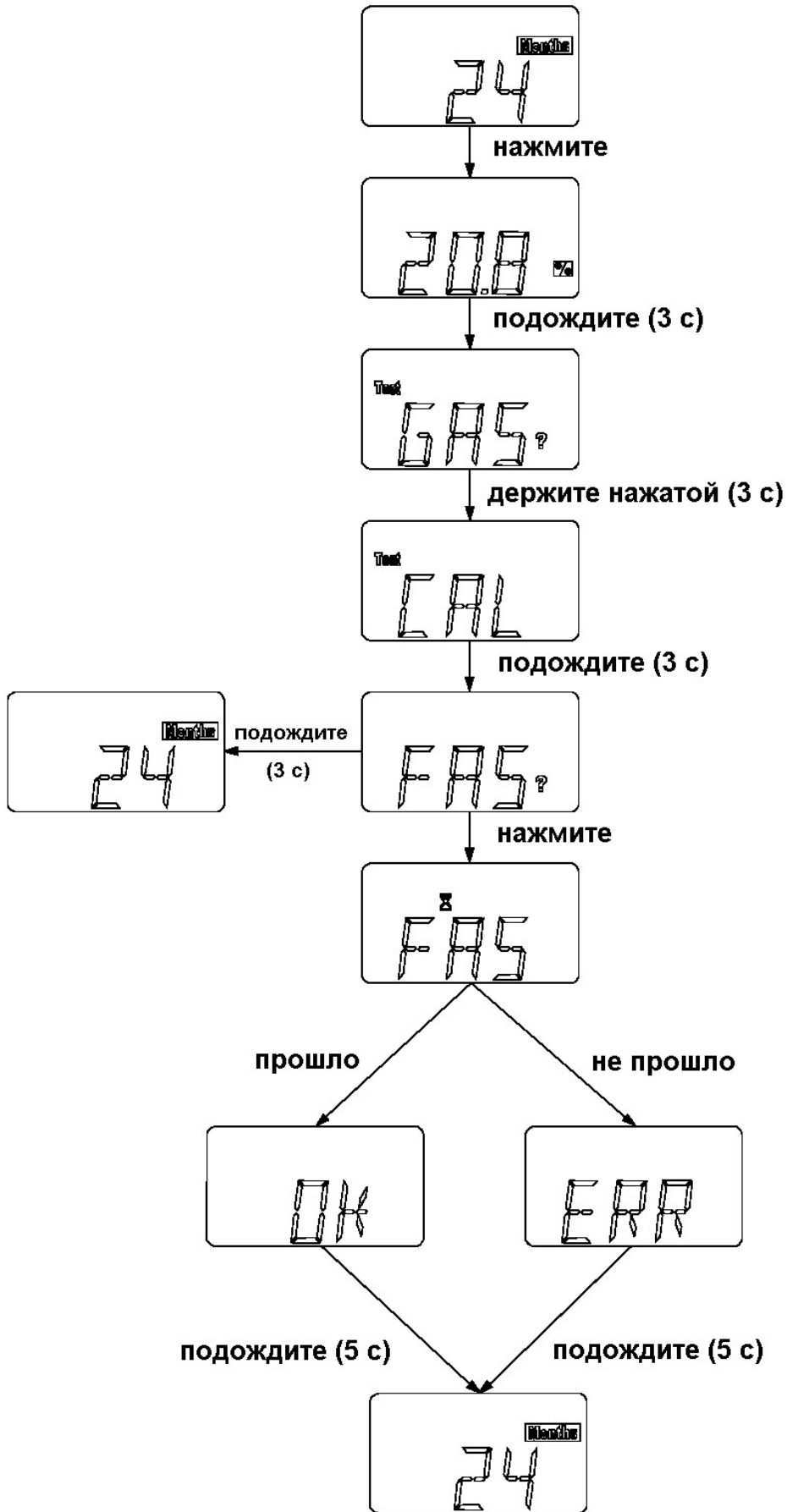
Рис. 9 Калибровка - Кислород
