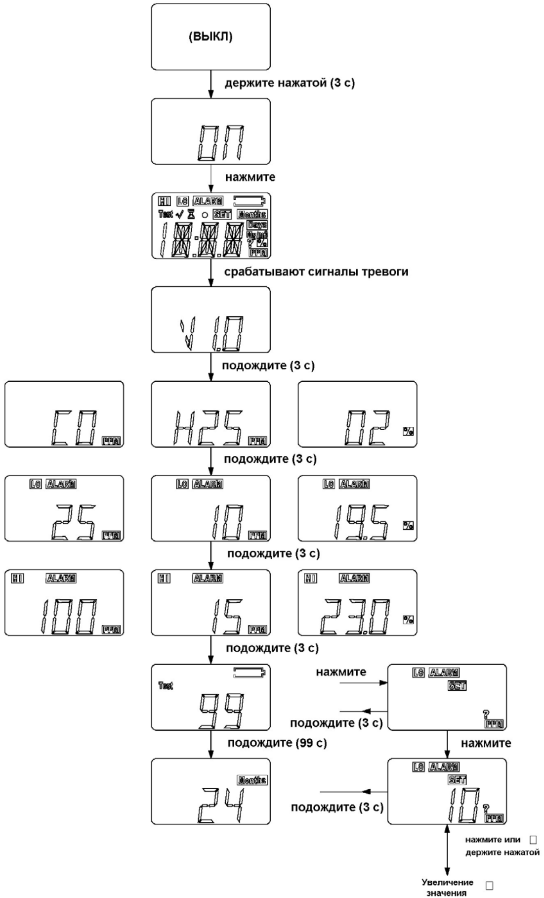
Рис. 4 Запуск сигнализатора
