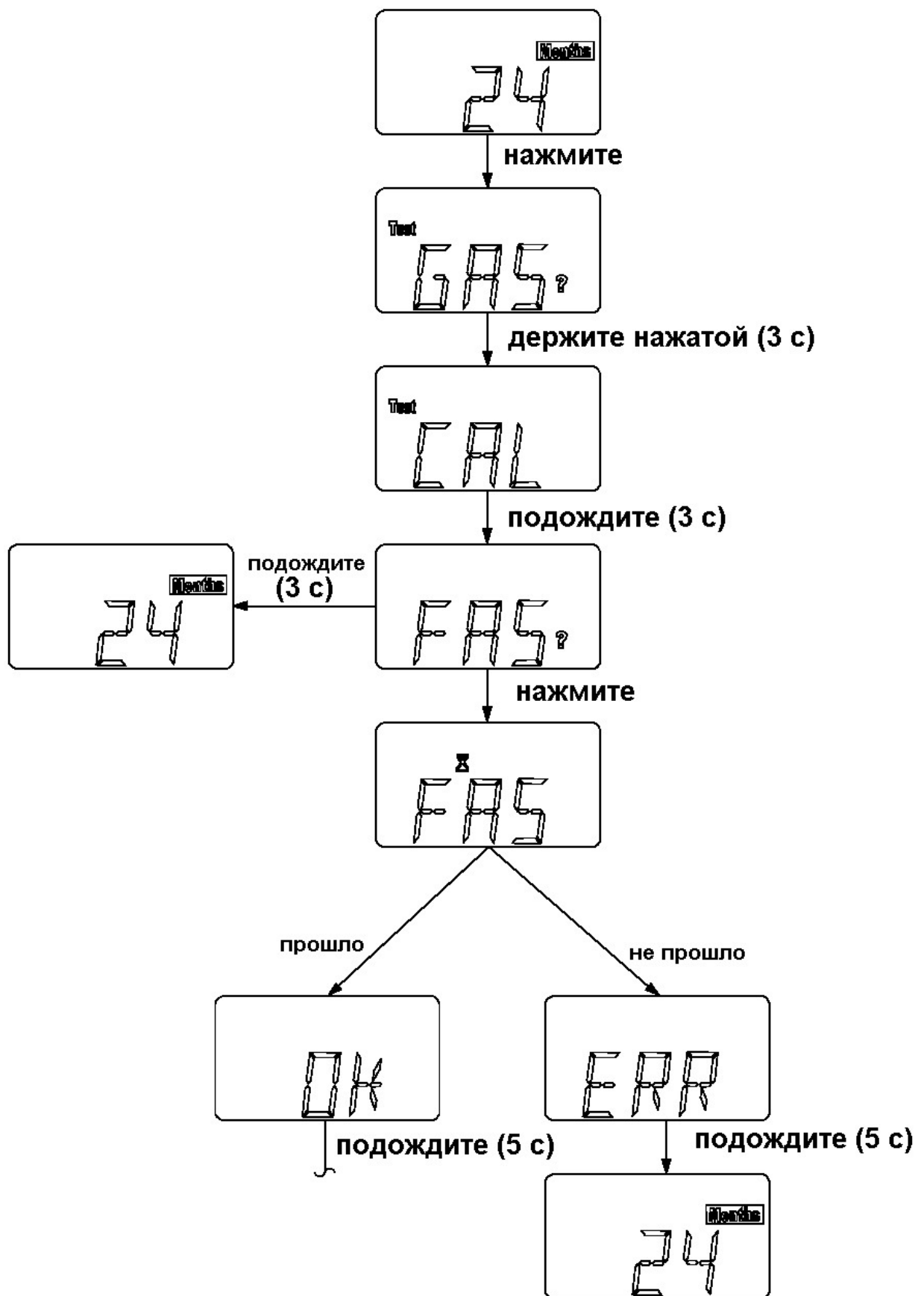
Рис. 7 Калибровка – Токсичные газы
