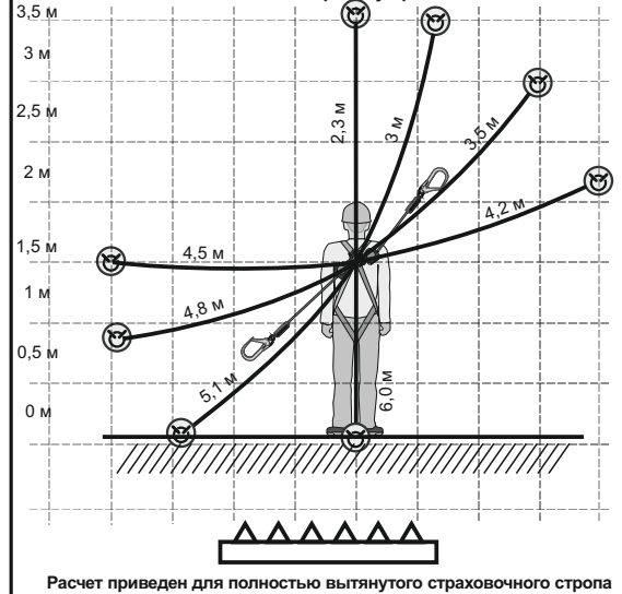
Рис. 9. Использование двухплечевой «НВ-02»
