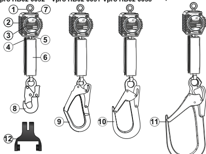
Рис. 1. Внешний вид, составные части и параметры врго НВ02 0052 врго НВ02 0051 врго НВ02 0058 врго НВ02 0258
