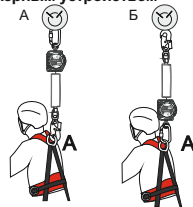
Рис. 3. Допустимые варианты присоединения блока «НВ-02» с анкерным устройством
