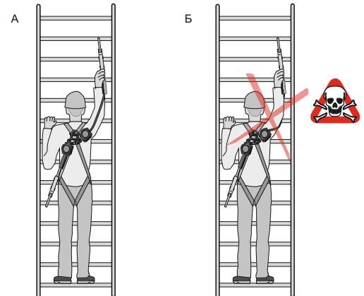
Рис. 9. Использование двухплечевой «НВ-02»
