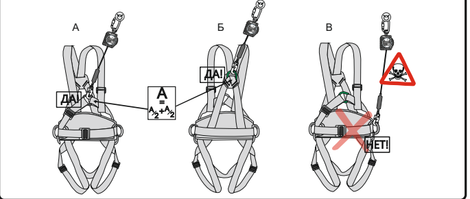
Рис. 4. Допустимые варианты соединения «НВ-02» с привязью
