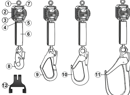
Рис. 1. Внешний вид, составные части и параметры
